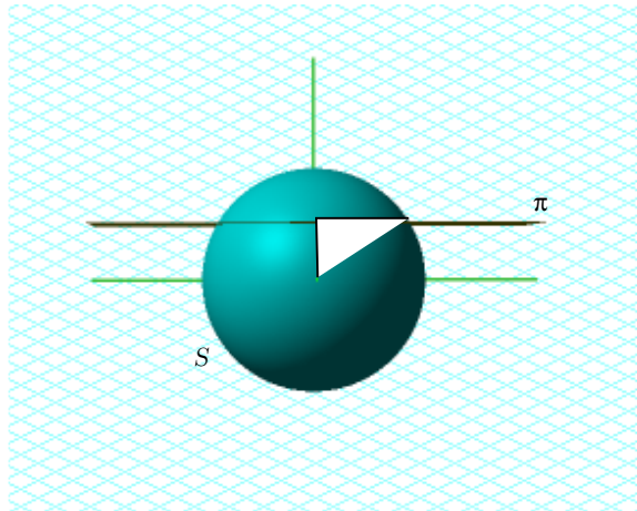
Fig.16. Il raggio della circonferenza \pi \cap S .
