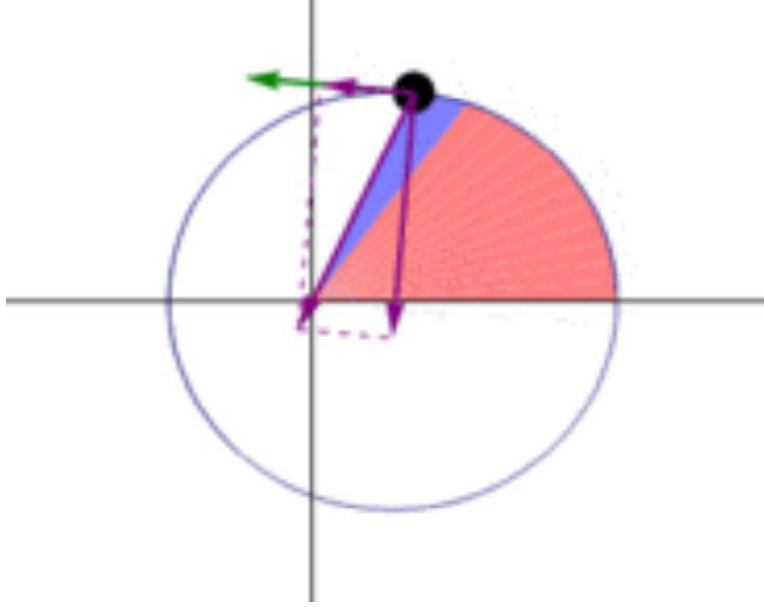
FIGURE 2. Illustrazione schematica del concetto di area spazzata dal raggio vettore che congiunge il centro di attrazione (che è posto nell'origine e può rappresentare, ad es., il Sole) con un punto materiale (ad es., un pianeta), che ruota attorno ad esso. Immagini prese dal sito http://en.wikipedia.org/wiki/Kepler's_laws_of_planetary_motion , dove sono reperibili altre informazioni riguardanti le leggi di Keplero.
