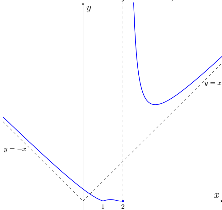
FIGURA 1. Grafico di f con a = 1 , b = 2 .
