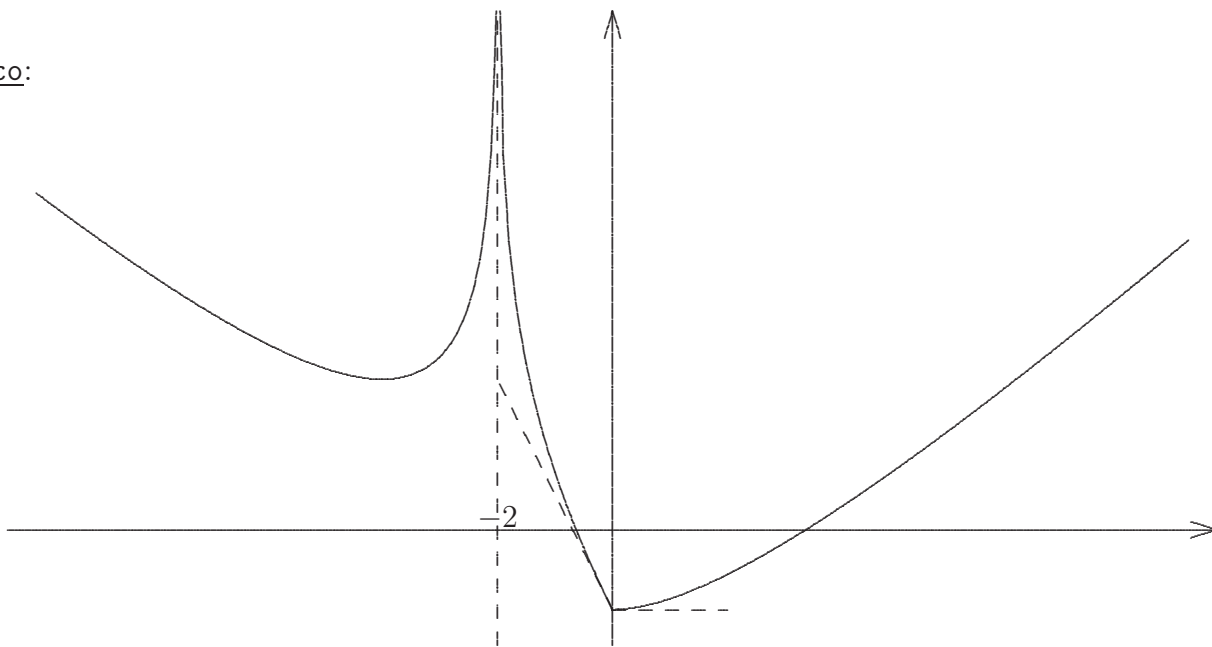
Figura 1: Tratteggiati l'asintoto verticale e le due tangenti nel punto di ascissa x = 0
