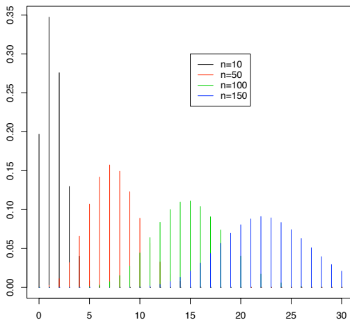
Distribuzione binomiale ( p=0.15 )
