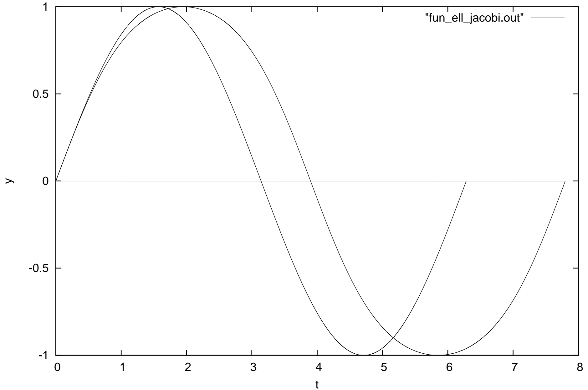
Confronto tra la funzione ellittica di Jacobi y=\text{sn}(t) e il seno trigonometrico y=\sin(t)
