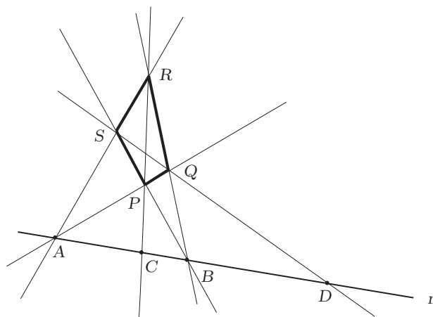
Il teorema del quadrangolo.
