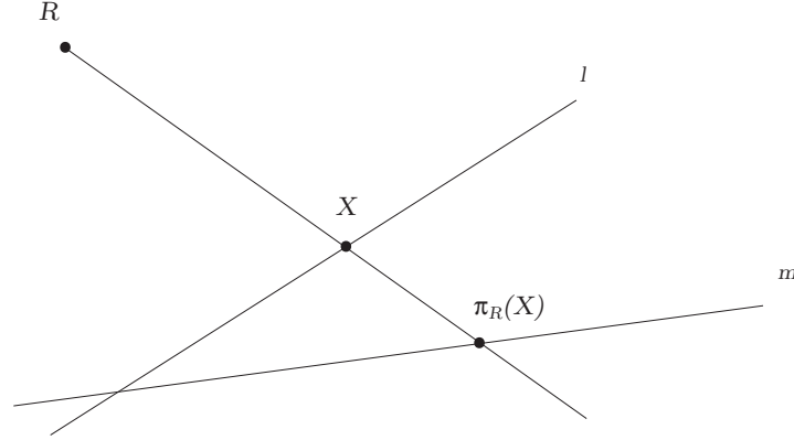
La prospettiva di centro R .
