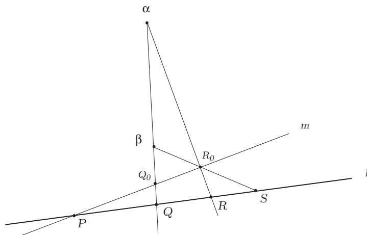
Costruzione della proiettività dell'Esempio 2.
