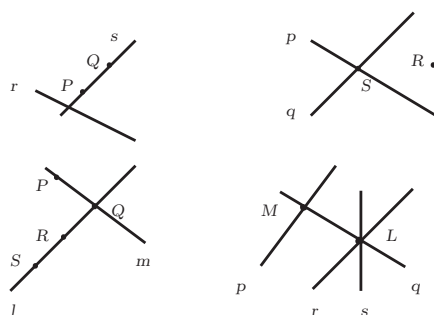
Esempi di configurazioni duali.
