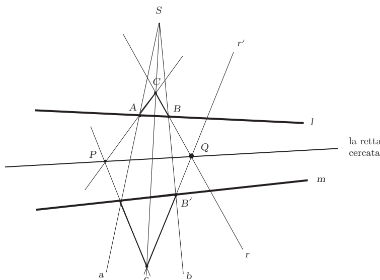
Applicazione del teorema di Desargues al Problema 1.
