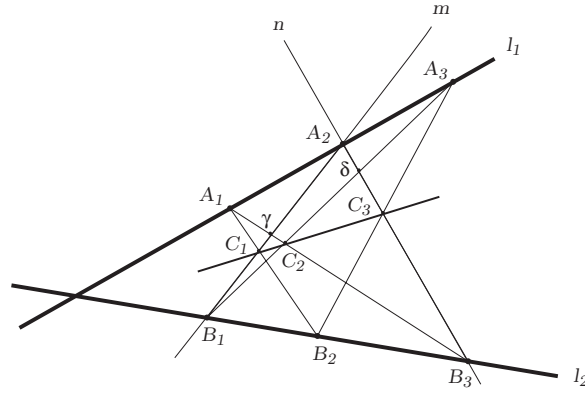
Il teorema di Pappo.
