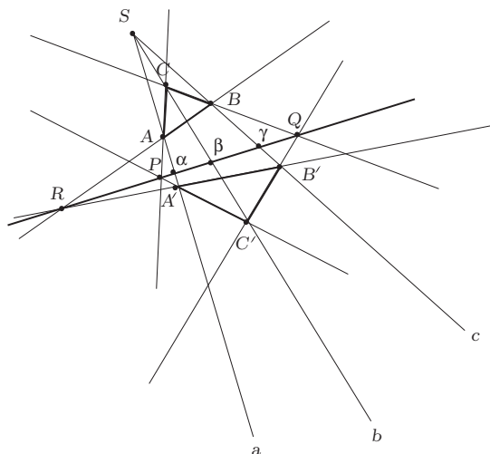
Il teorema di Desargues.
