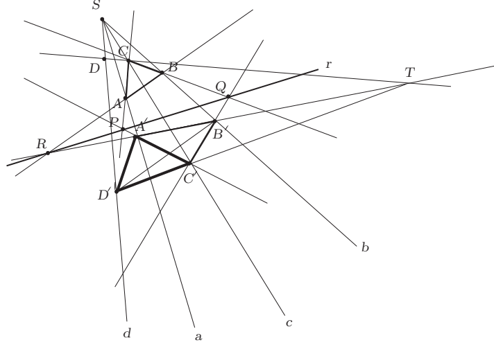
Applicazione del teorema di Desargues al Problema 2.
