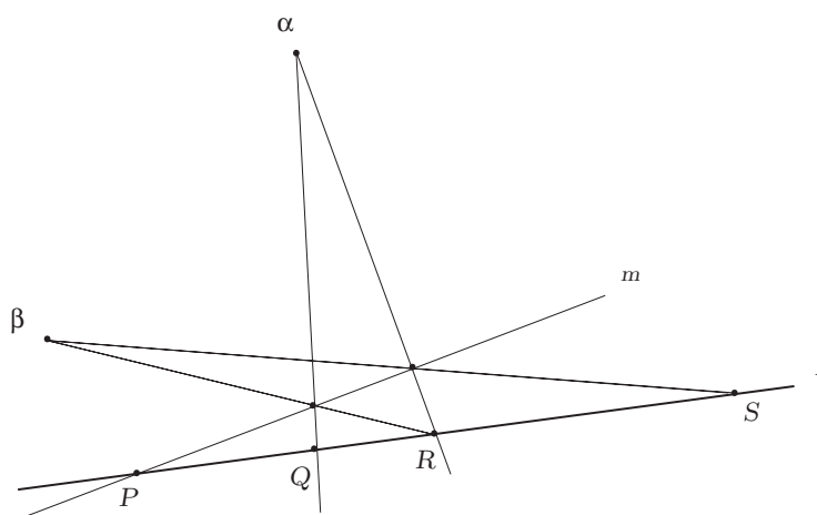
Costruzione della prospettività dell'Esempio 1.
