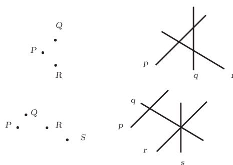
Esempi di configurazioni duali.
