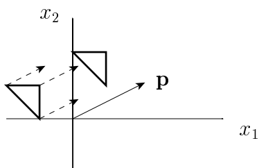
Figure 1: La traslazione T_{\mathbf{p}} .
