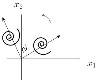
Figure 2: La rotazione R_{\phi} .
