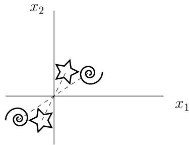
Figure 5: La riflessione rispetto all'origine R_\pi = S_0 \circ S_{\pi/2} .
