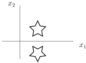
Figure 4: La riflessione rispetto all'asse delle ascisse S_0 .
