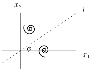
Figure 3: La riflessione S_{\phi} .
