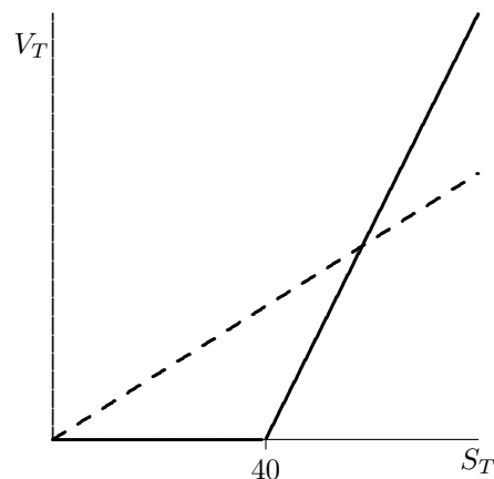
Figura 1.3 Grafico del valore dell'investimento V_T in funzione del prezzo S_T ; in tratteggio, il valore di V_T nella prima strategia.
